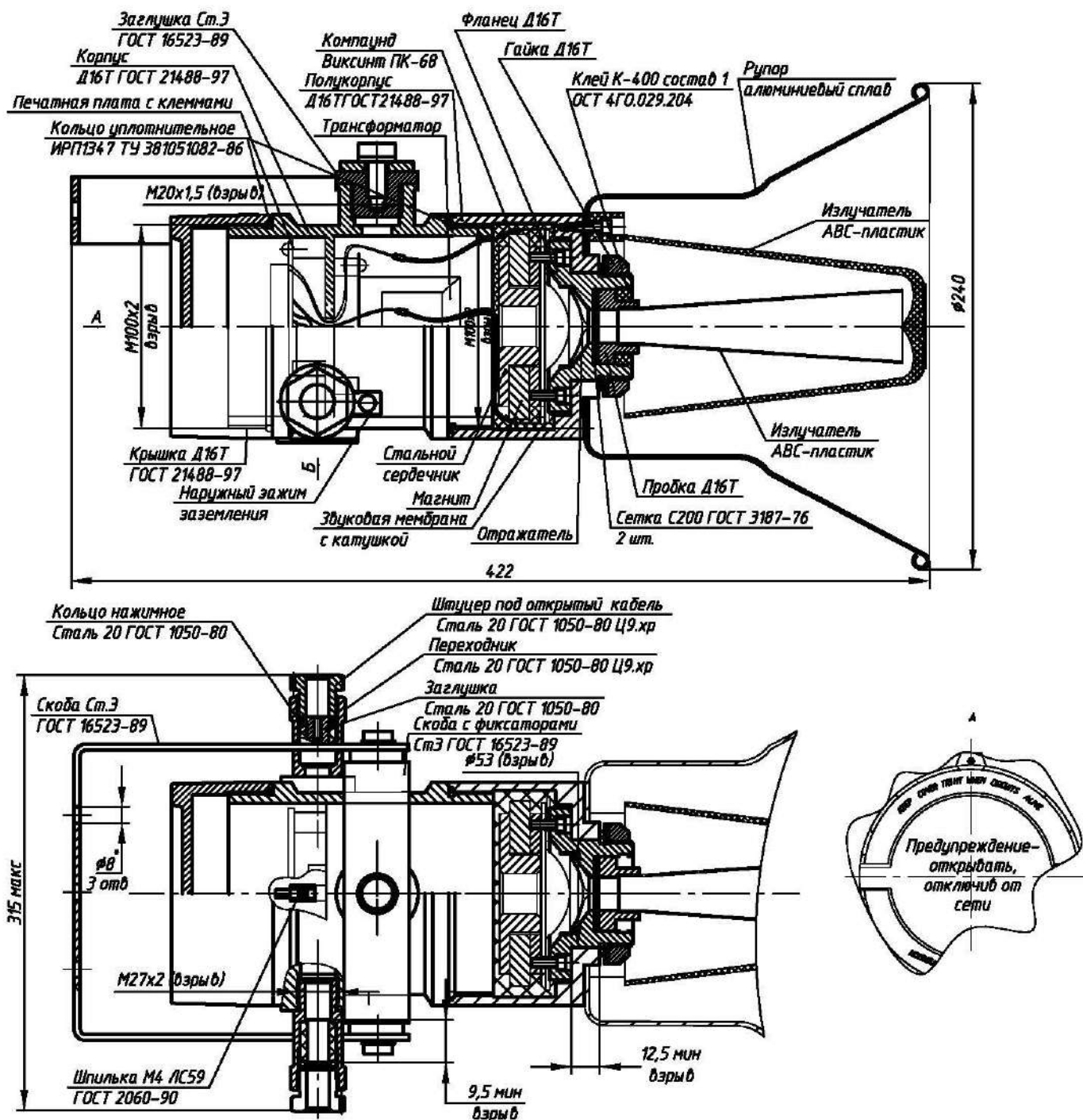
Рис. Г.1 Габаритный чертёж громкоговорителя ГРВ-25А, совмещённый с чертежом средств взрывозащиты (вариант 2 по КД 908.2370.00.000)
