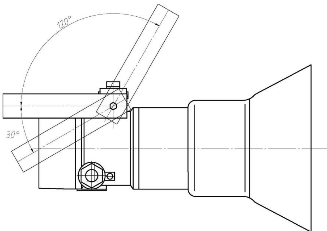
Рис. Г.2 Положение громкоговорителя ГРВ-25А при эксплуатации
