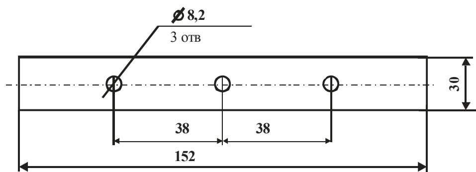
Рис. Г.3 Размеры отверстий на скобе громкоговорителя ГРВ-25А
