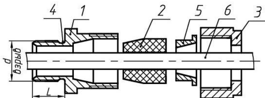
Рис. В.3.б – Порядок сборки кабельного ввода К для открытой прокладки небронированного кабеля:
