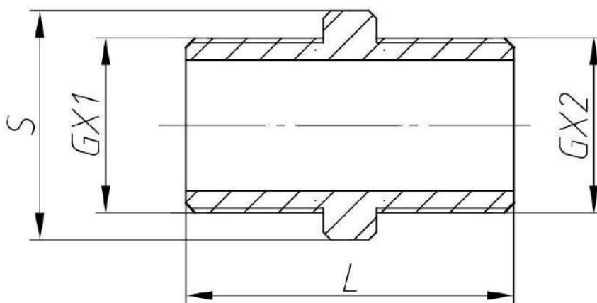
Рис. В.4.в – Ниппель компании Valtec Размеры см в таблице В.4.б ниже. При исполь- зовании учитывать внутренний диаметр ниппеля и диаметр ка- беля
